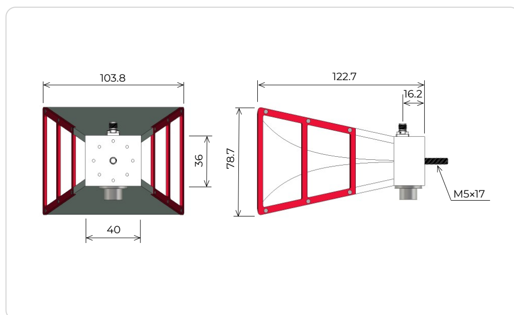
Antenna
