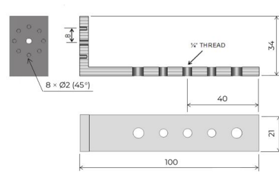
Flange
